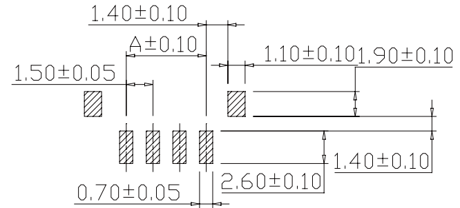
P.C.B LAYOUT
